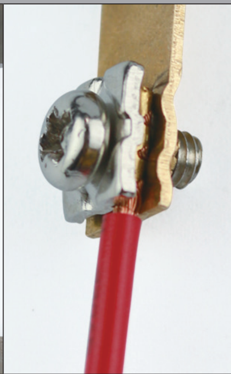
Klemmen-Detail
